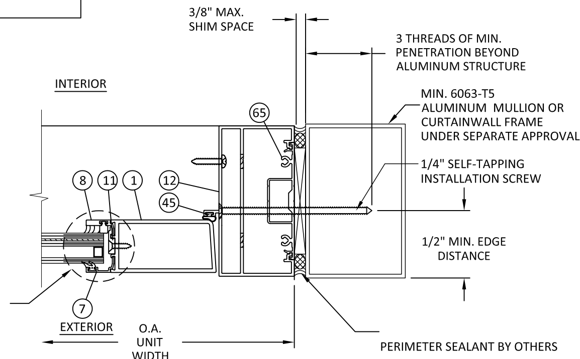
H HORIZONTAL SECTION 4 DOOR JAMB - ALUMINUM STUD
