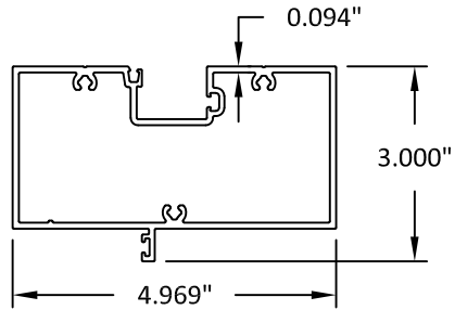
13 TRANSOM BAR (MONO)
